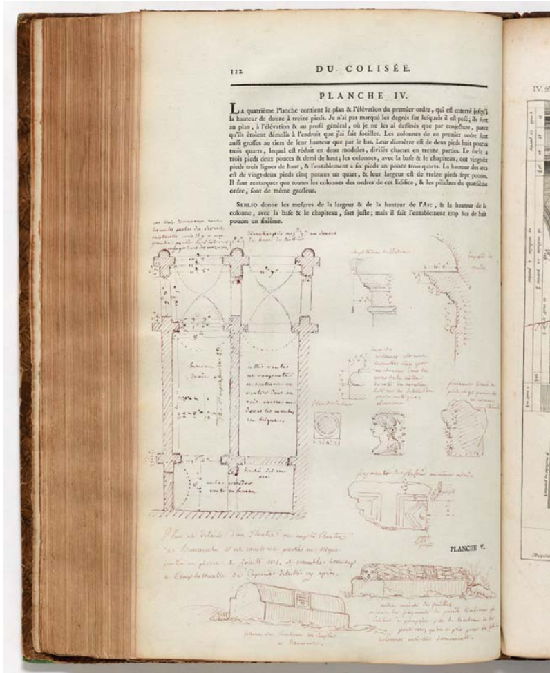
Fig. 27 (below) Plan et details d'un Theatre ou amph Theatre a Benevent
